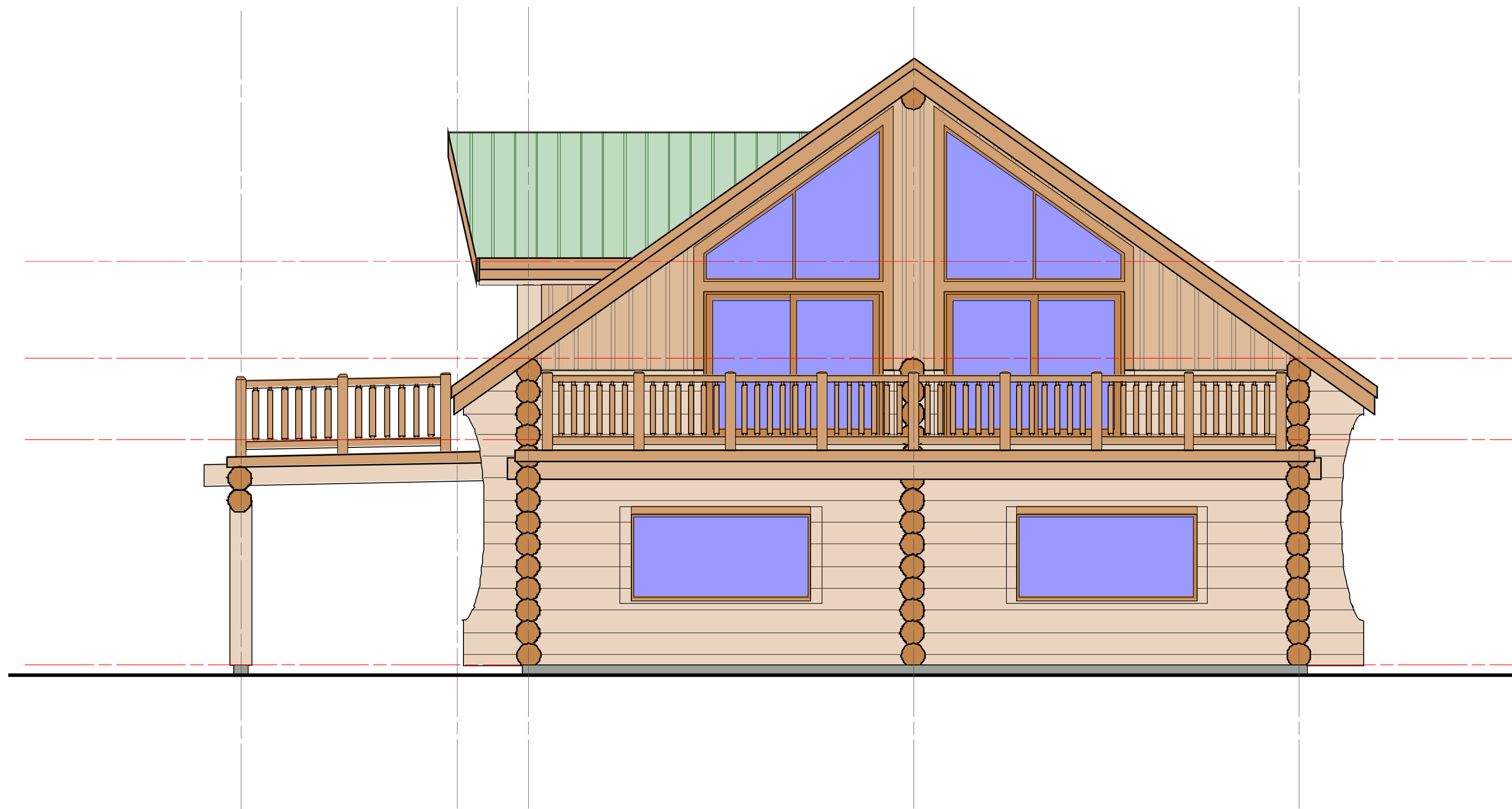
SOUTH ELEVATION SCALE: 1:50
